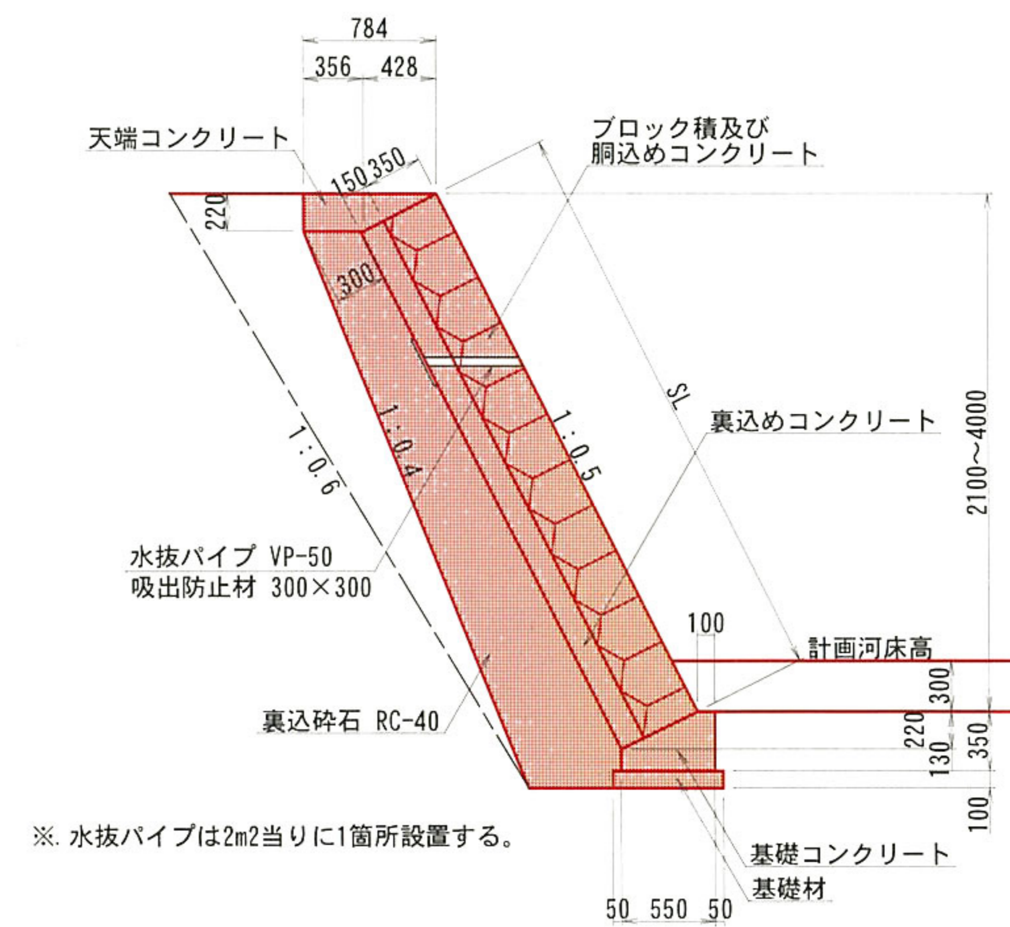
ブロック積護岸断面図 S=1:30
