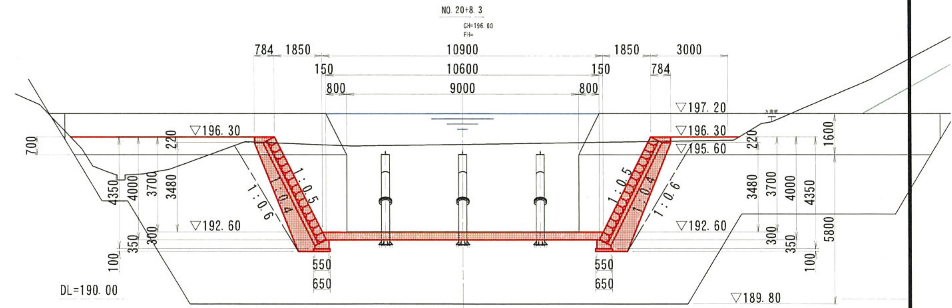
ぶって沢第1号堰堤垂直壁正面図 S=1:100
