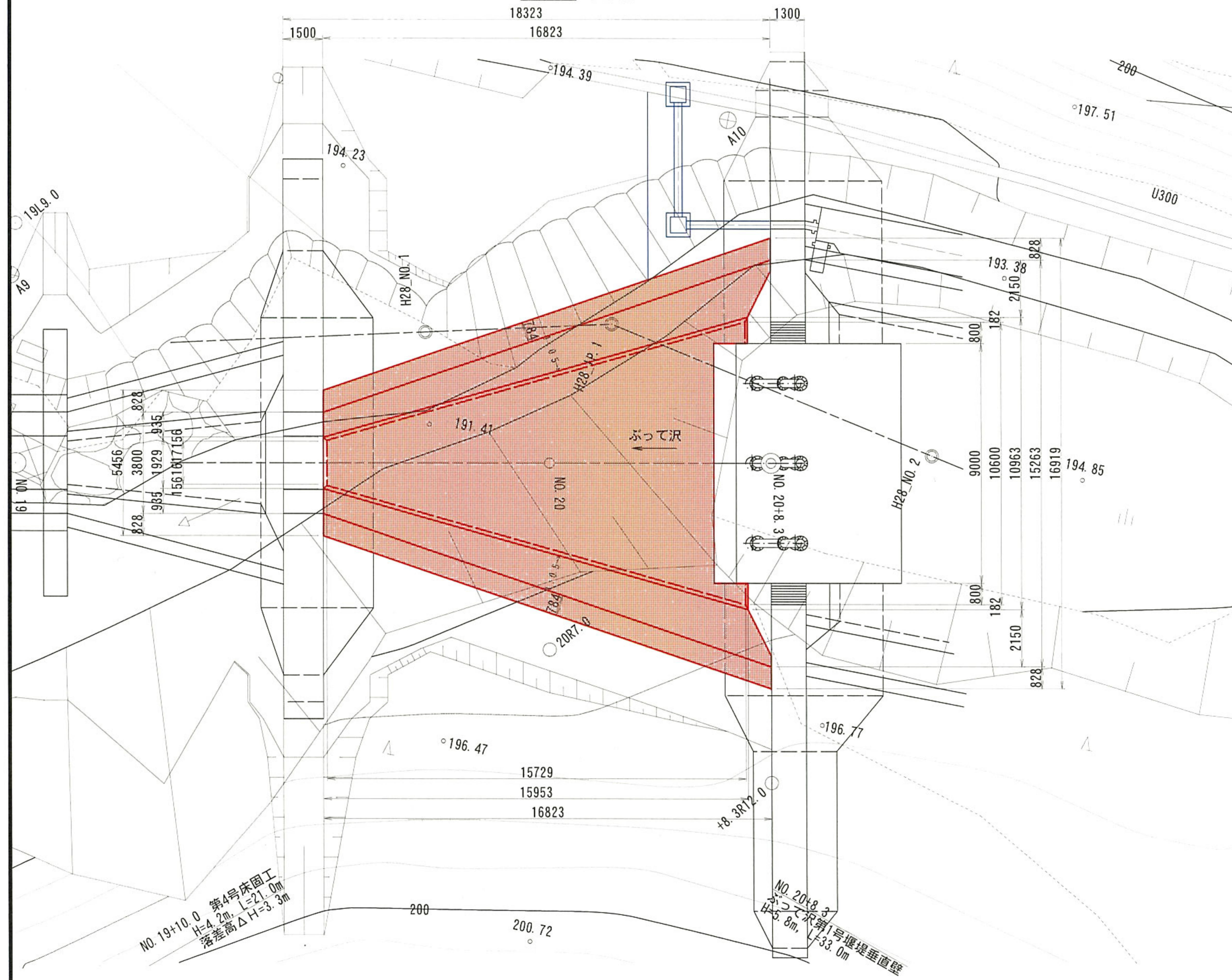
平面図 S=1:100
