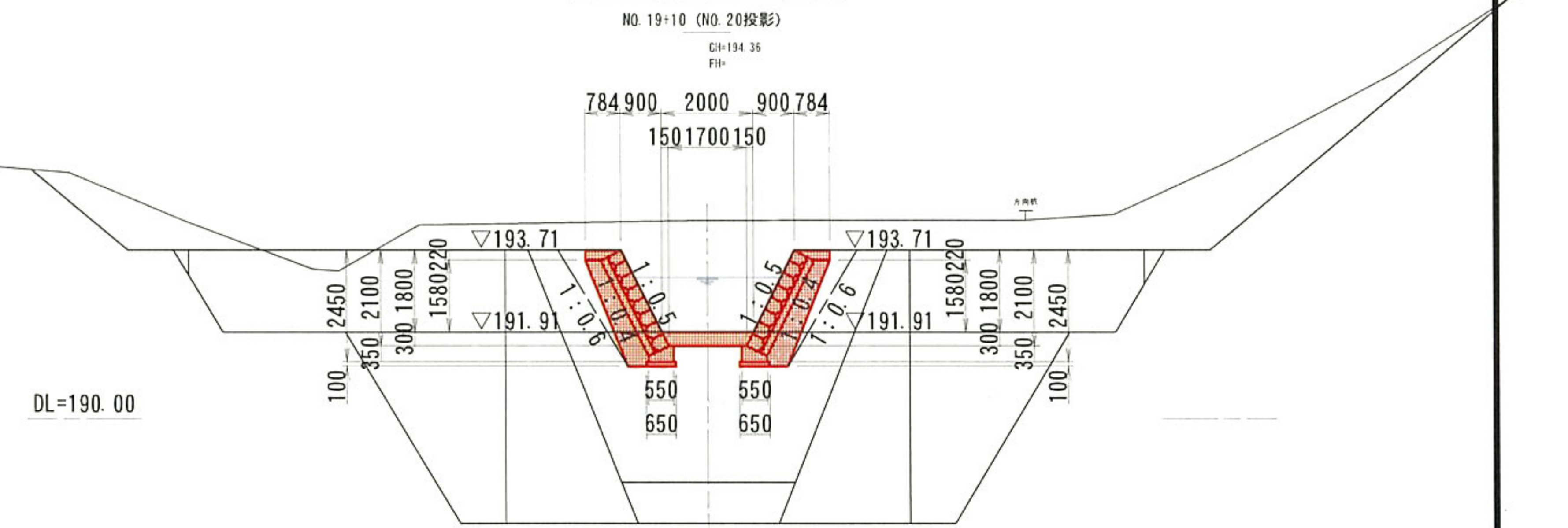
第4号床固工正面図 S=1:100
